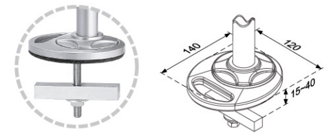
FA-227 Grommet Type
