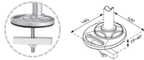
FA-52X-1 Grommet Type
