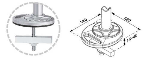
FA-225 Grommet Type
